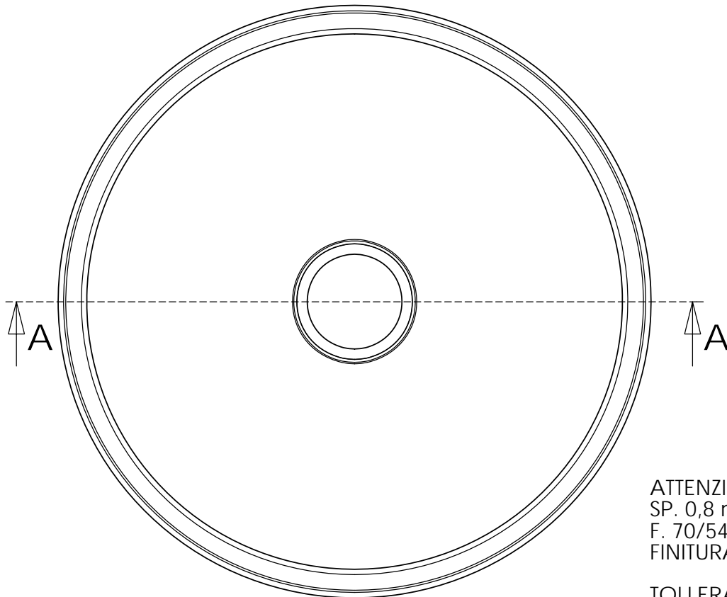
SEZIONE A-A
