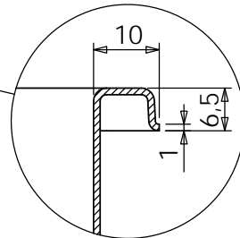
DETTAGLIO BORDO
